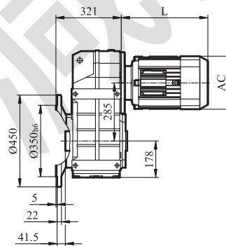
GFH/GFHZ/GFHF97输出轴
