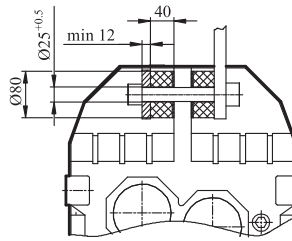
GFA97-T
