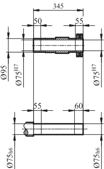
GFH/GFHZ/GFHF97输出轴
