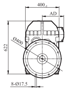
GFV/GFVZ/GFVF97输出轴
