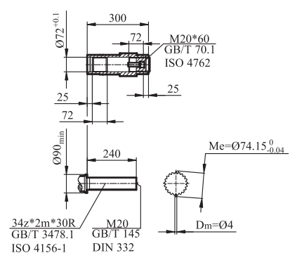
GFV/GFVZ/GFVF97输出轴
