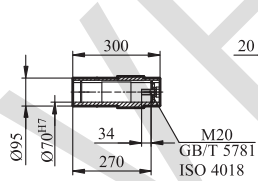
GFA/GFAZ/GFAF97输出轴
